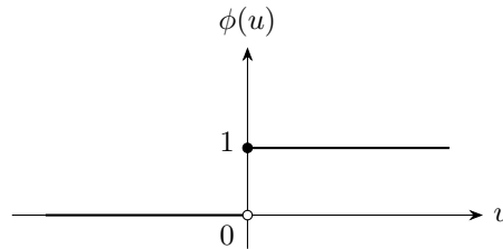
Figura 2.3: Función de activación escalón unitario.
